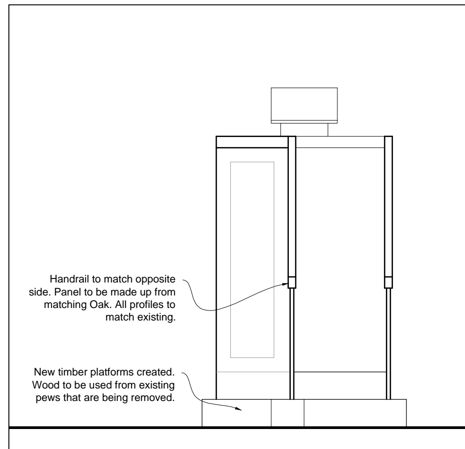
ELEVATION B 1:20
